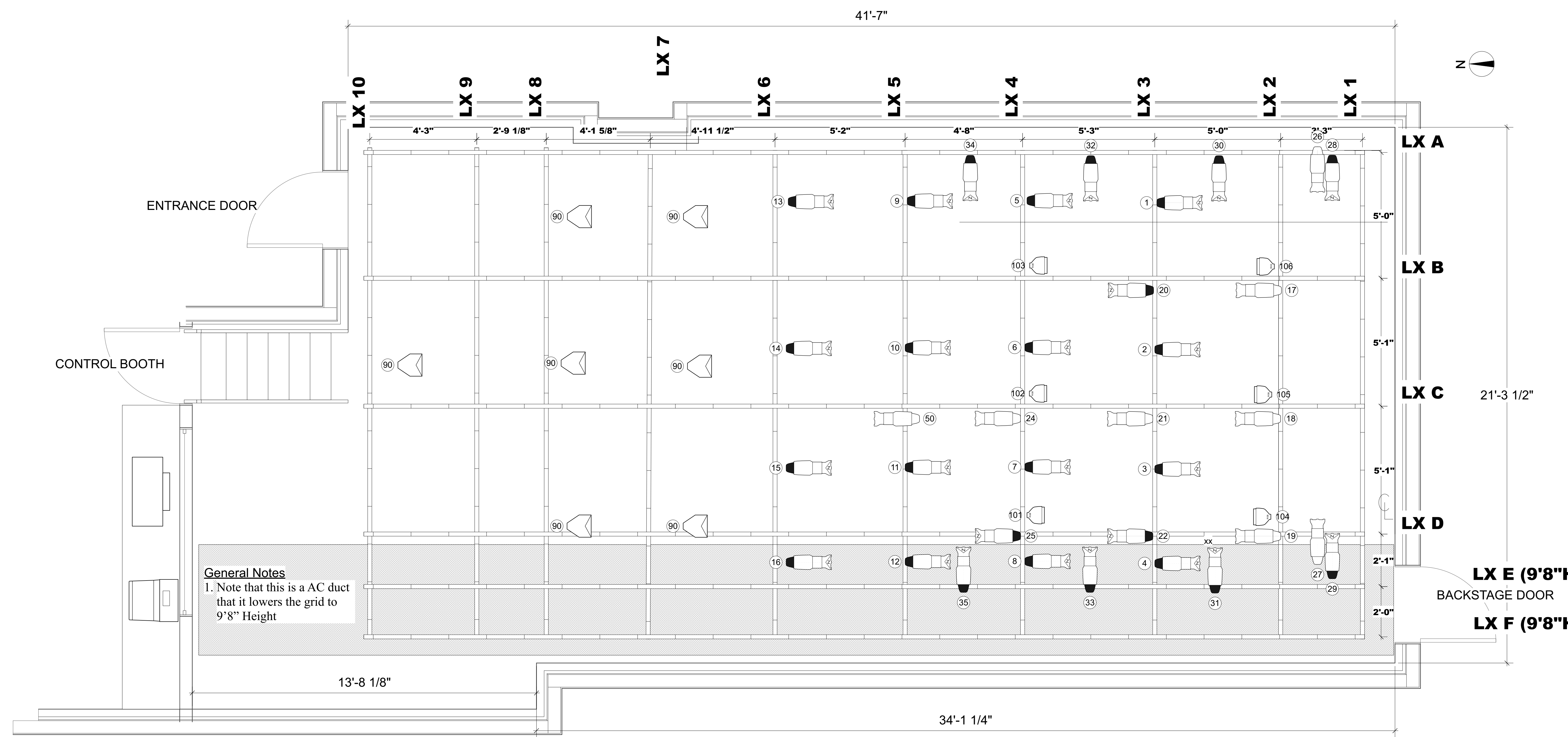
1 Top View Scale: 1/2" = 1'-0"
